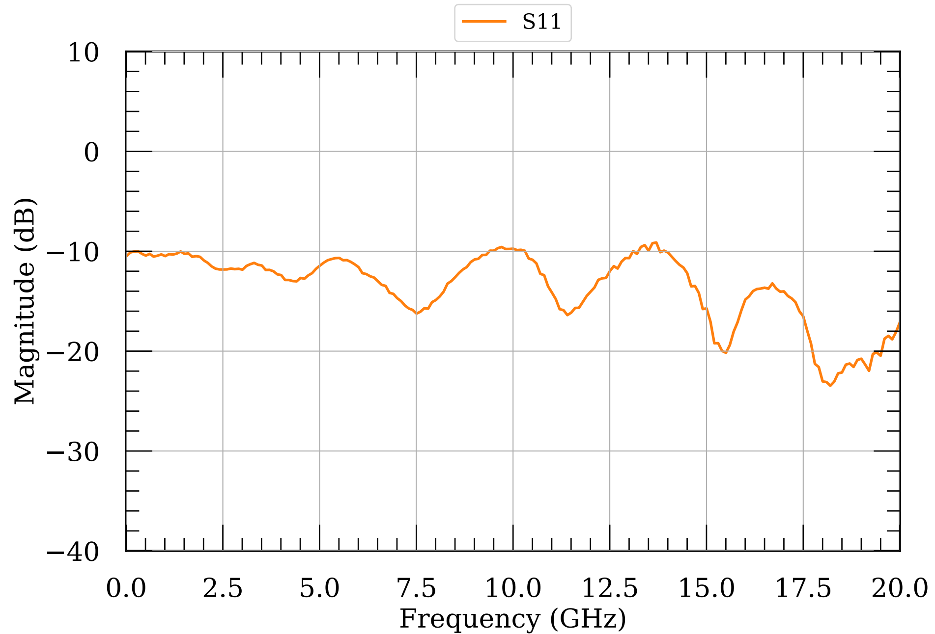
LNA S-params module041v2
